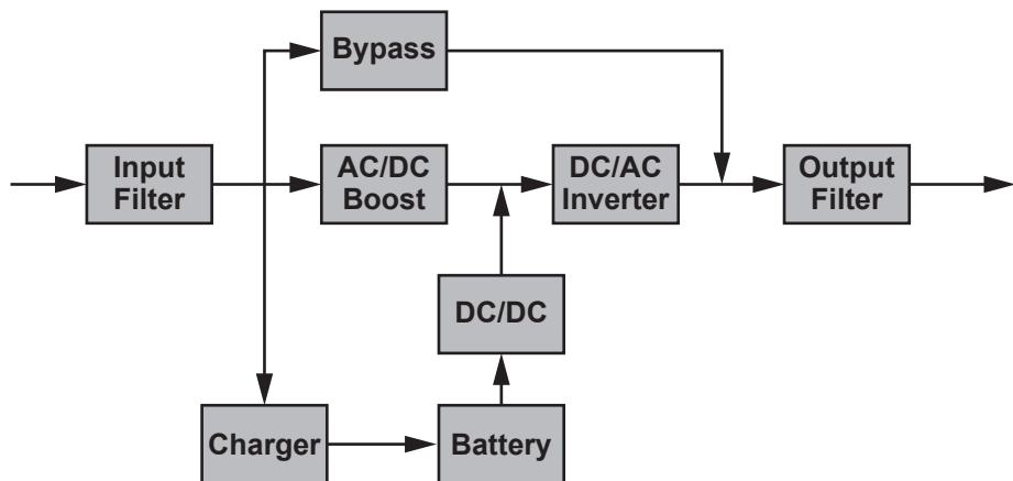
Блок-схема ИБП
