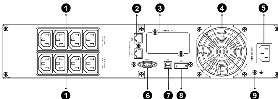
Задняя панель модели Smart Winner II 2000E
