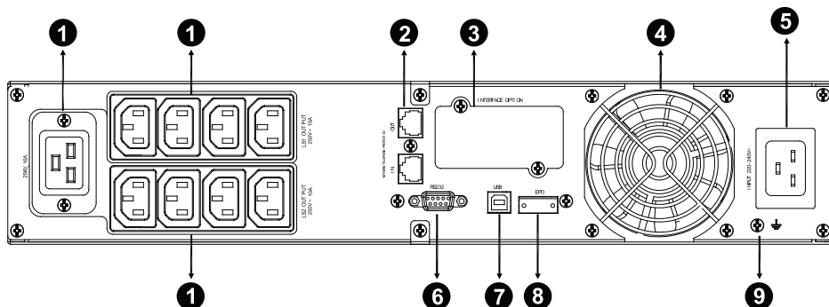
Задняя панель модели Smart Winner II 3000
