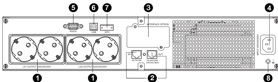
Задняя панель модели Smart Winner II 1500 EURO
