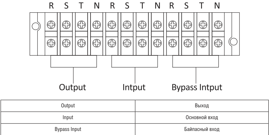
Схема подключения клеммной колодки Innova RT 33 20K Tower
