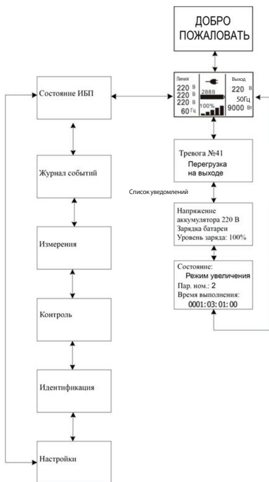
Рис. 5-14 Структура главного меню
